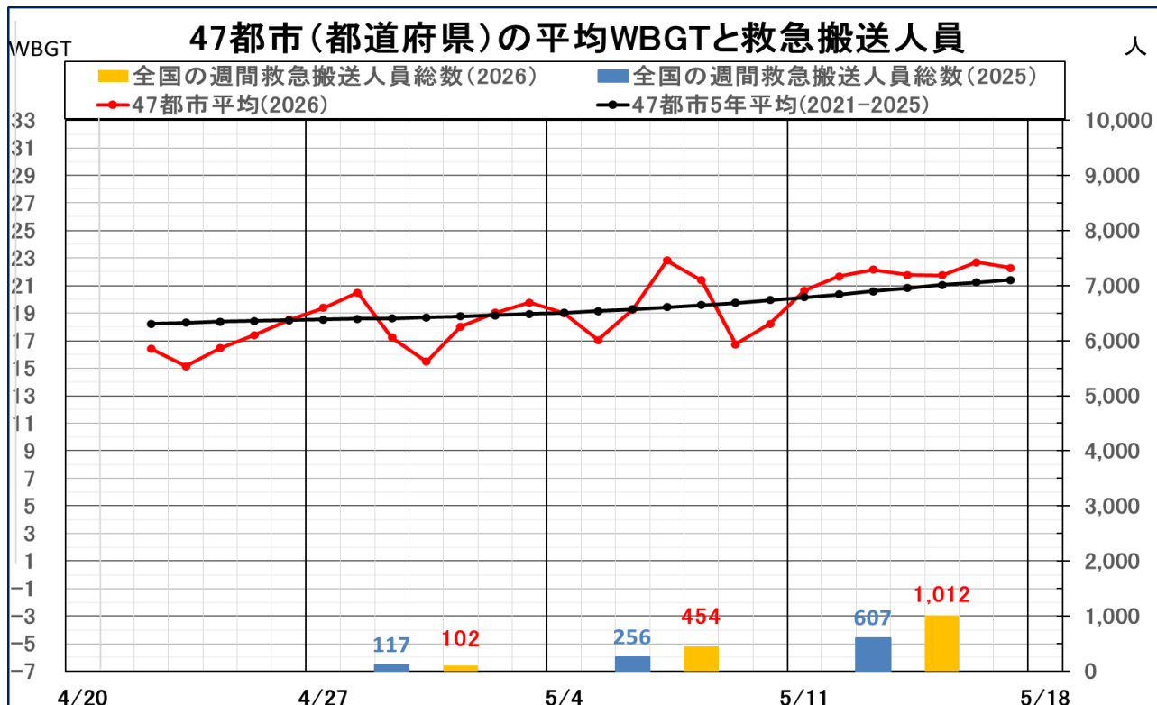
図1 全国47都市の平均日最高暑さ指数(WBGT)状況と救急搬送人員(全国)の動向
