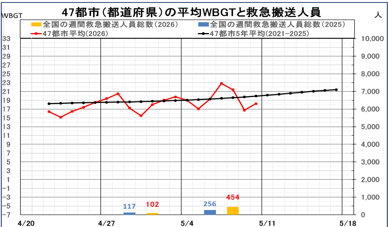
図1 全国47都市の平均日最高暑さ指数(WBGT)状況と救急搬送人員(全国)の動向
